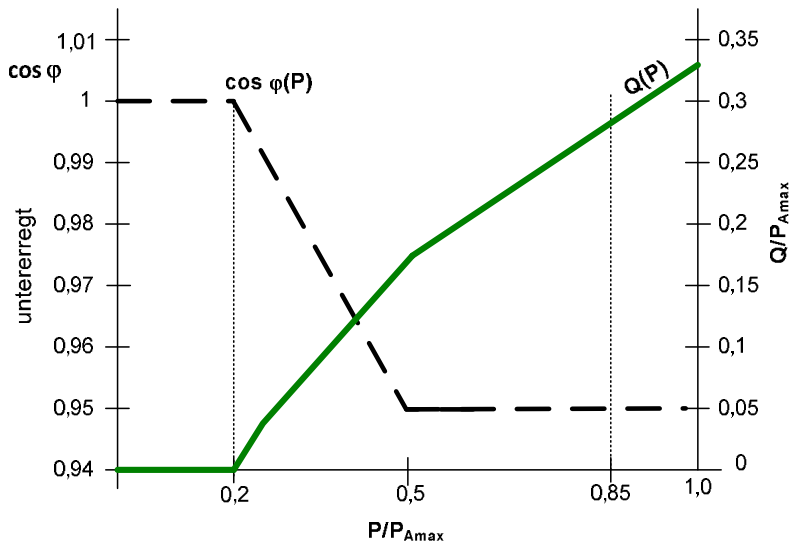
Bild 3 Q = f(P/P_{Amax}) -Kennlinie für Erzeugungsanlagen mit P_{Amax} \geq 135 kW und Anschluss in den Umspannungsbereichen Königsbrück, Kamenz, Zescha, Kleinsaubernitz, Niesky, Görlitz und Weinhübel
