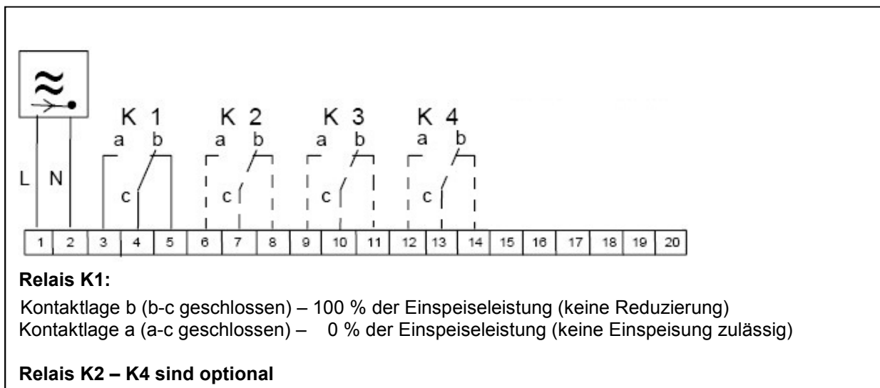
Bild 1 Anschlussschema des FRE
